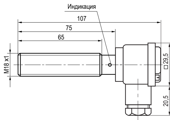
Габаритный чертеж.
