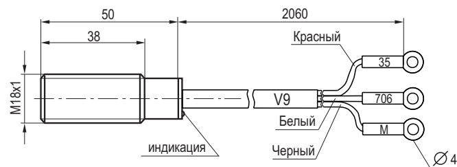
Габаритный чертеж
