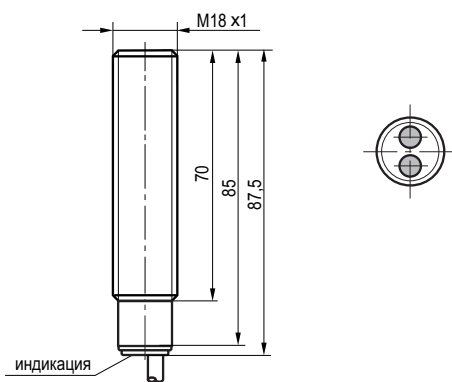
Габаритный чертеж
