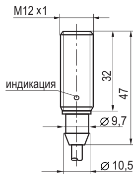
Габаритный чертеж
