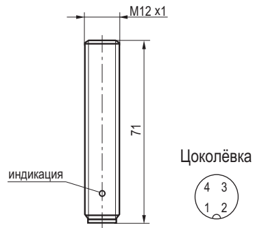
Габаритный чертеж
