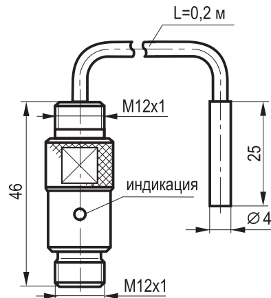
Габаритный чертеж
