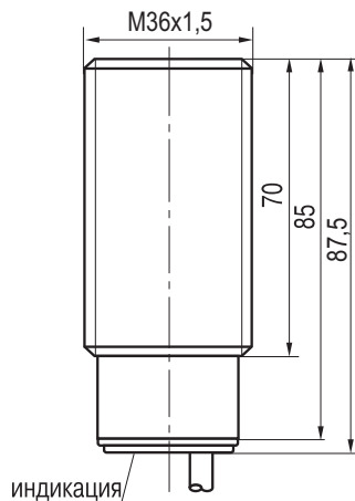
Габаритный чертёж
