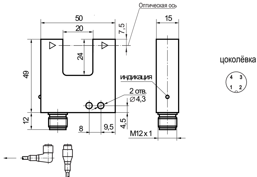
Габаритный чертеж
