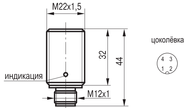
Габаритный чертеж
