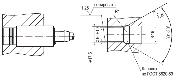
Схема монтажа
