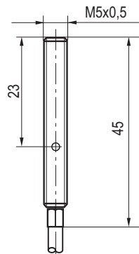
Габаритный чертеж
