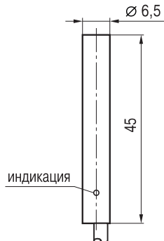
Габаритный чертеж
