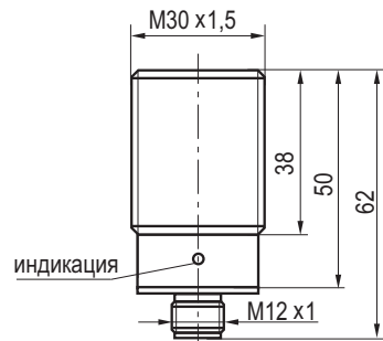
Габаритный чертеж
