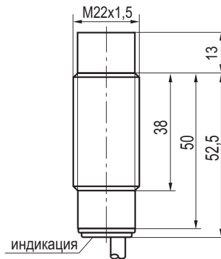
Габаритный чертеж
