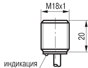
Габаритный чертеж
