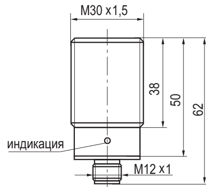
Габаритный чертеж
