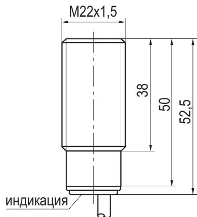
Габаритный чертеж
