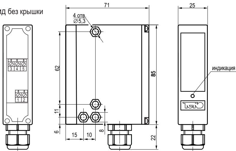
Габаритный чертеж.
