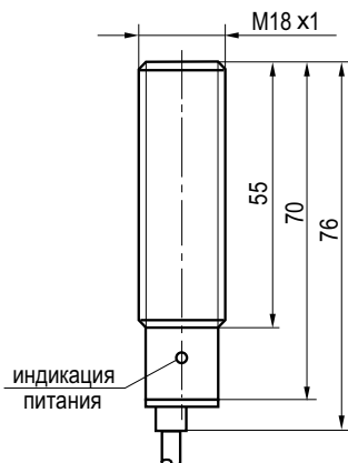
Габаритный чертеж
