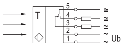
Схема подключения
