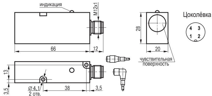
Габаритный чертеж
