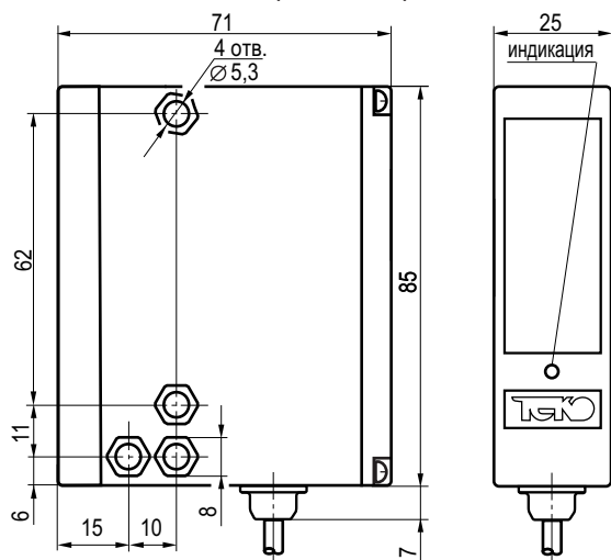
Габаритный чертеж
