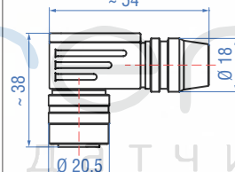
Розетка, угловая, 7 конт., M16 Артикул № 560 779
