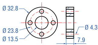
Кольцевой магнит OD33 Артикул № 201 542-2
