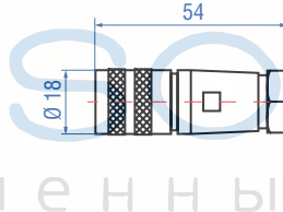
Розетка, прямая, 7 конт., M16 Артикул № 370 624
