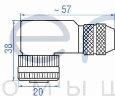
Розетка, угловая, 8 конт., M12 Артикул № 370 699
