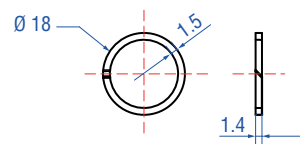
Опорное кольцо Артикул № 561 115
