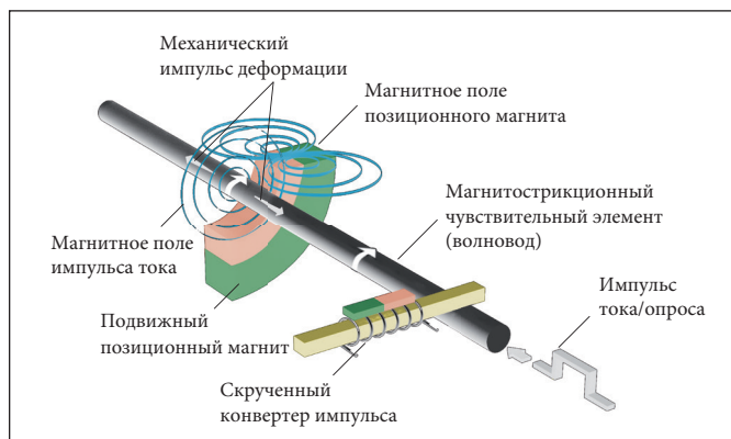
Рис. 1: Магнитострикционный принцип
