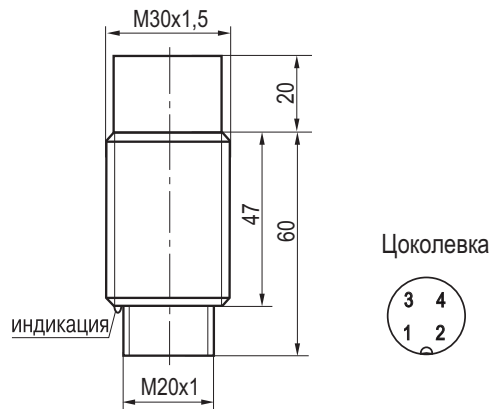
Габаритный чертеж
