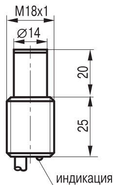
Габаритный чертеж
