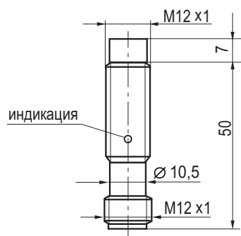
Габаритный чертеж
