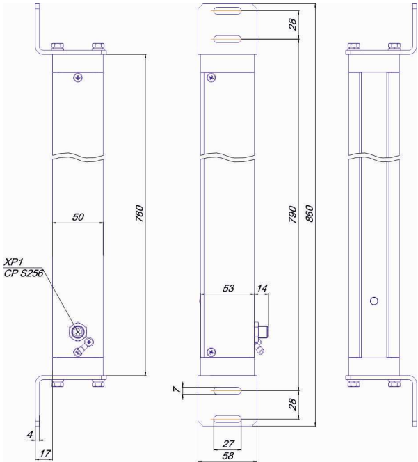
Габаритный чертеж Стойка излучателей (приемников)
