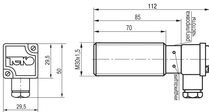
Габаритный чертеж
