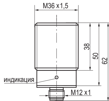
Габаритный чертеж
