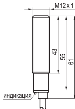
Габаритный чертеж
