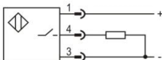
PNP NO
