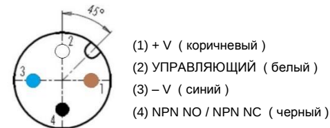
Выход NPN NO / NC для датчика с разъемом M12, 4-конт., штекер
