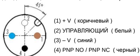
Выход PNP NO / NC для датчика с разъемом M12, 4-конт., штекер
