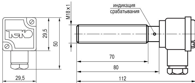
Габаритный чертеж.
