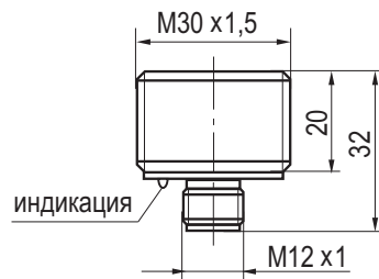
Габаритный чертеж
