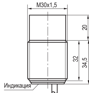
Габаритный чертеж
