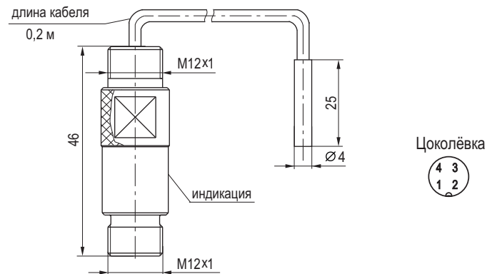
Габаритный чертеж
