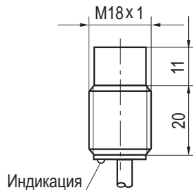
Габаритный чертеж
