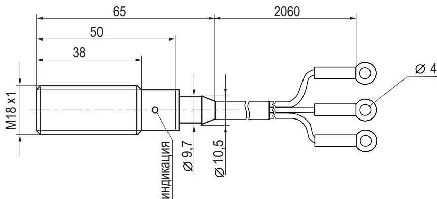
Габаритный чертеж
