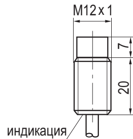
Габаритный чертеж
