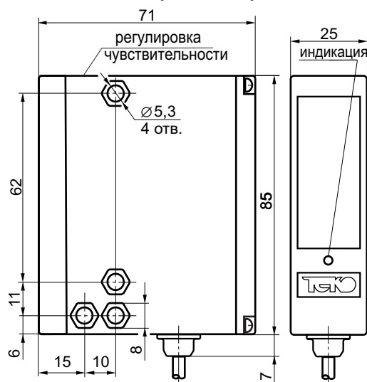
Габаритный чертеж.
