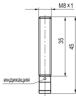
Габаритный чертеж
