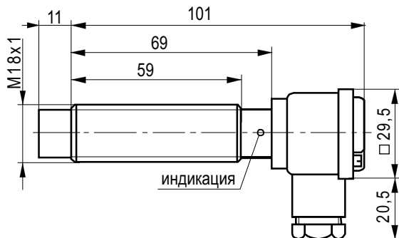
Габаритный чертеж
