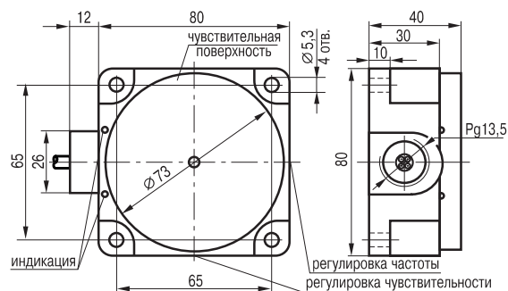
Габаритный чертеж
