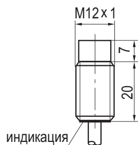
Габаритный чертеж
