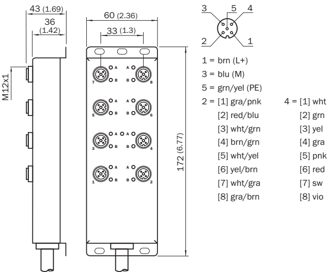
Габаритный чертеж (Размеры, мм)
