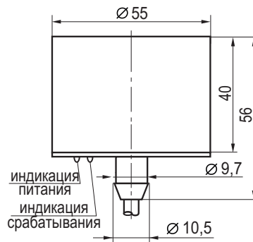
Габаритный чертеж
