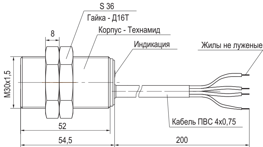
Габаритный чертеж
