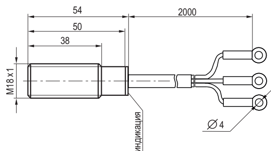
Габаритный чертеж
