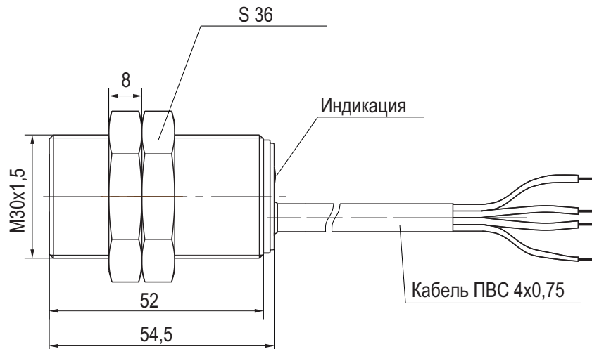
Габаритный чертеж
