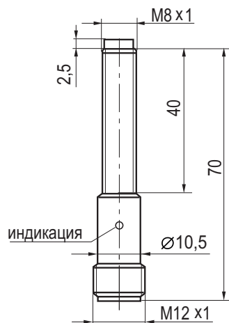
Габаритный чертеж
